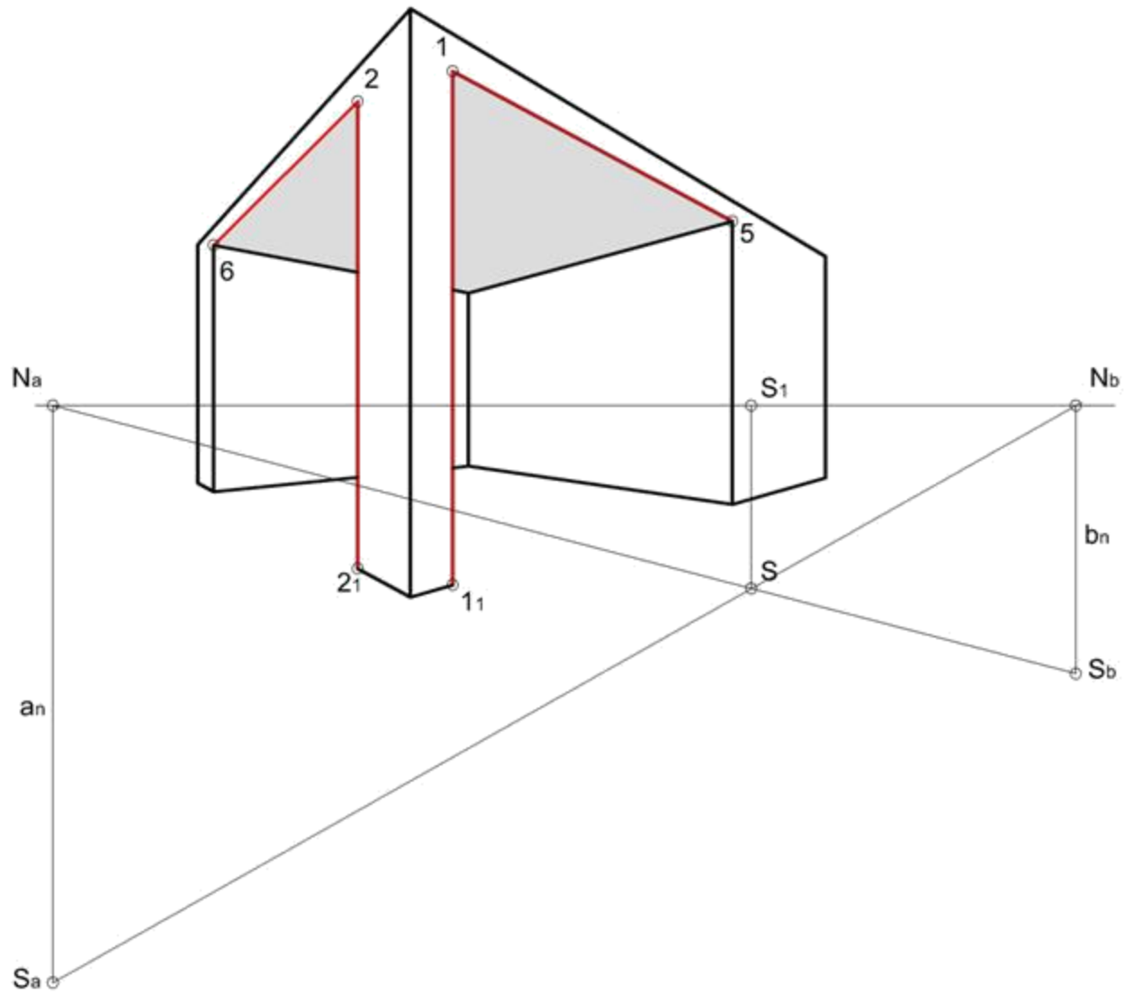
Пример конструисања бачене сенке од сунца у перспективи „са угла“
