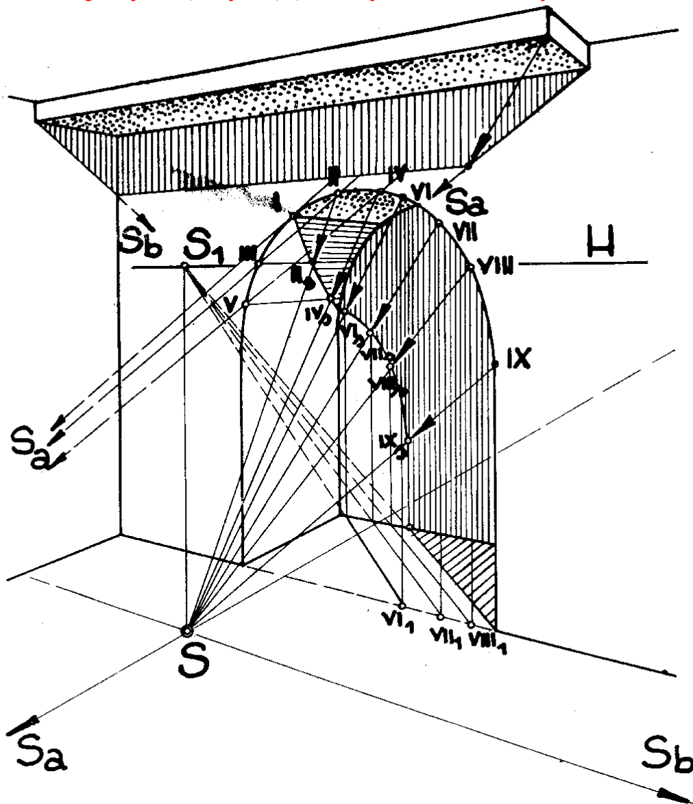
Пример конструисања бачене сенке од сунца у перспективи „са угла“
