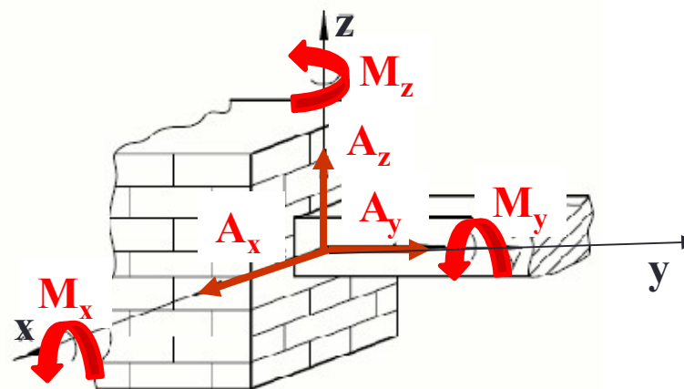
Uklještenje u prostoru
