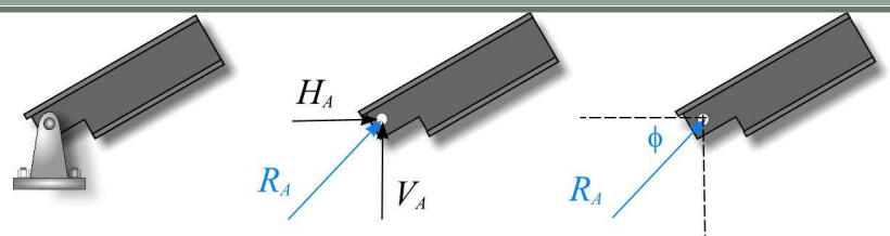
Cilindrični zglob i nepokretan oslonac
