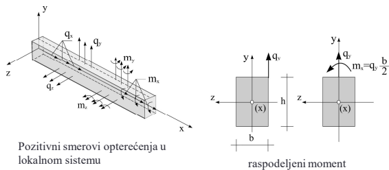
raspodeljeni moment
