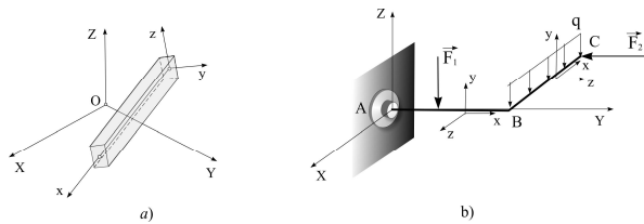
Štap u globalnom i lokalnom sistemu
