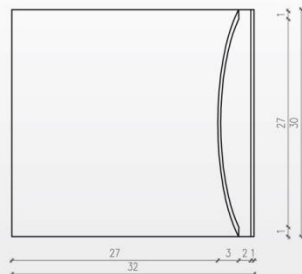
изглед постоља за таблет, p=1:5
