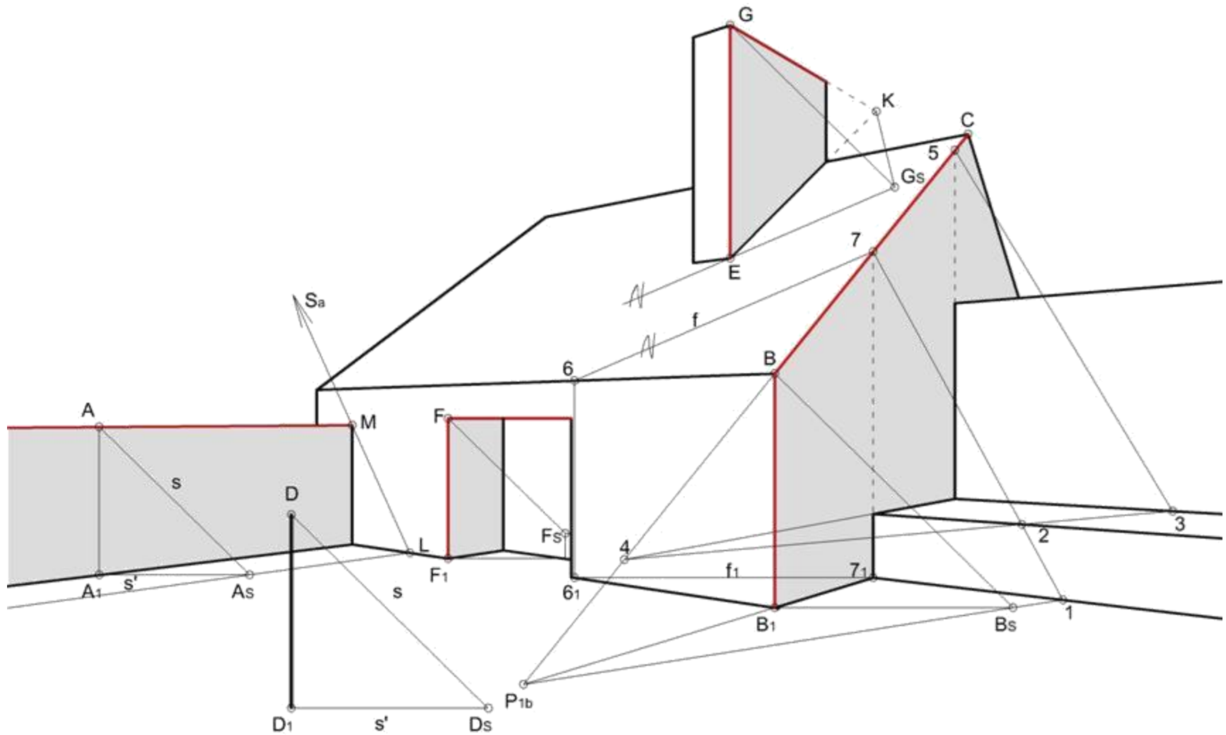
Пример конструисања бачене сенке од сунца у перспективи „са угла“
