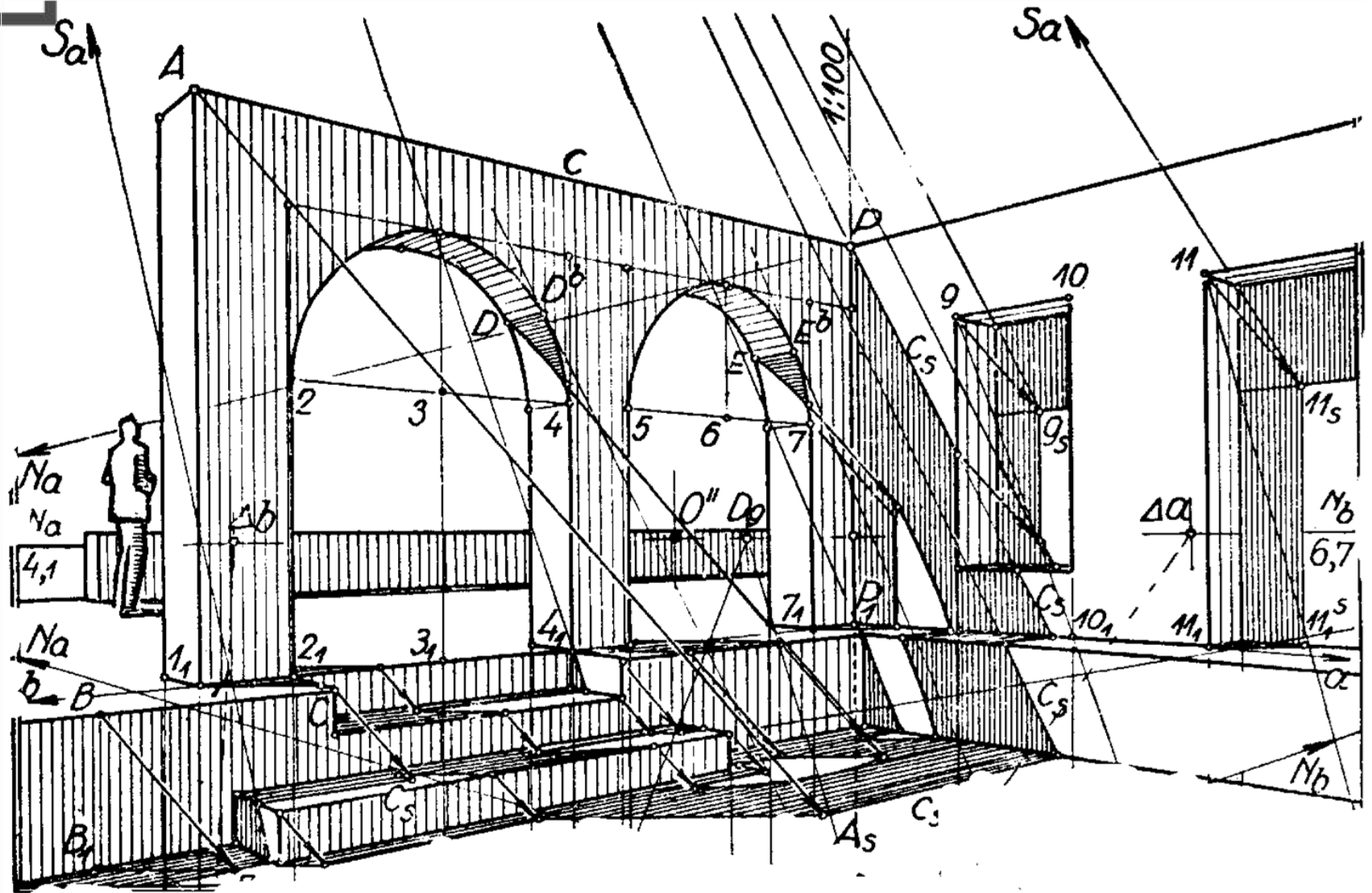
Пример конструисања бачене сенке од сунца у перспективи „са угла“
