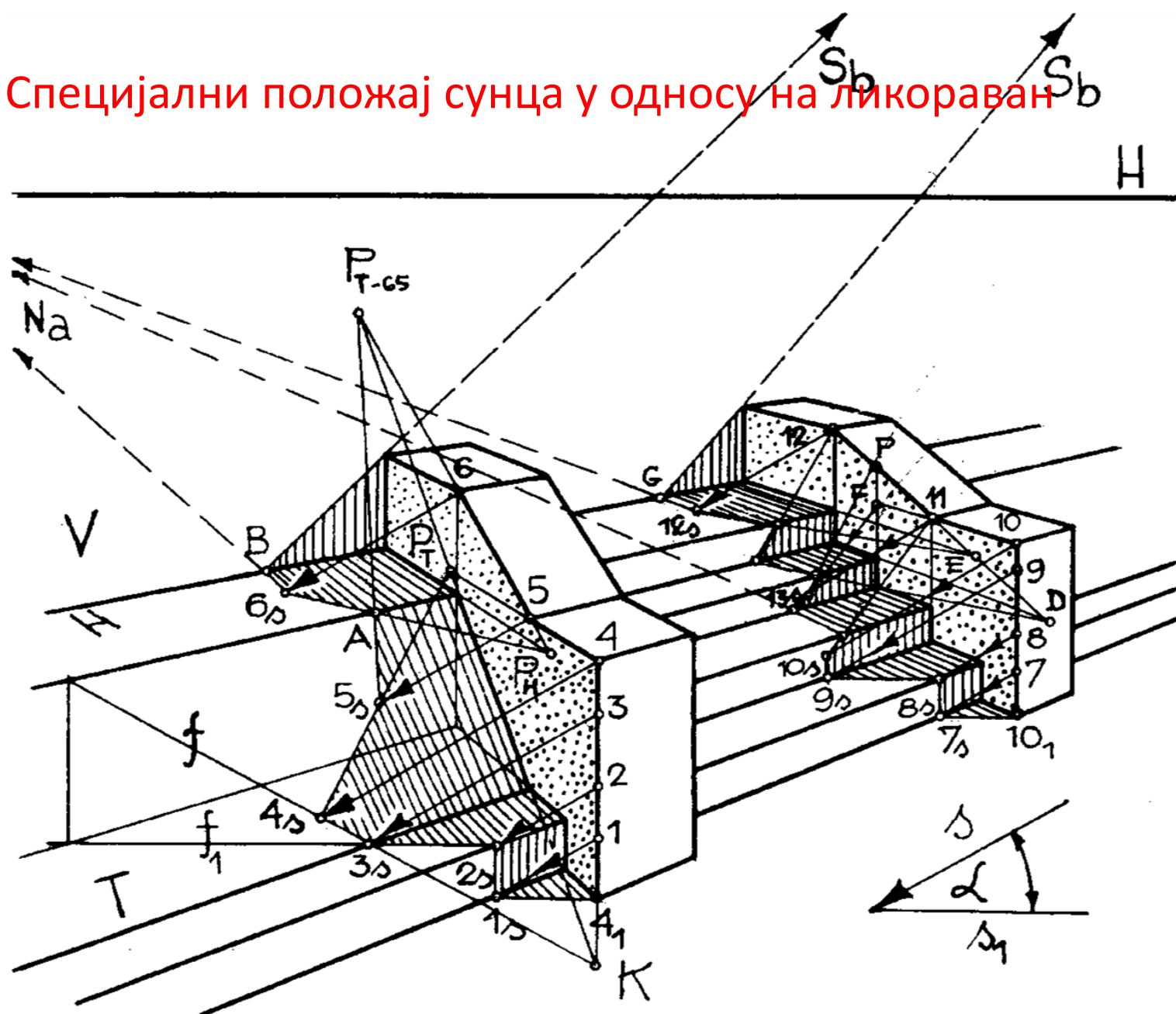
Пример конструисања бачене сенке од сунца у перспективи „са угла“
