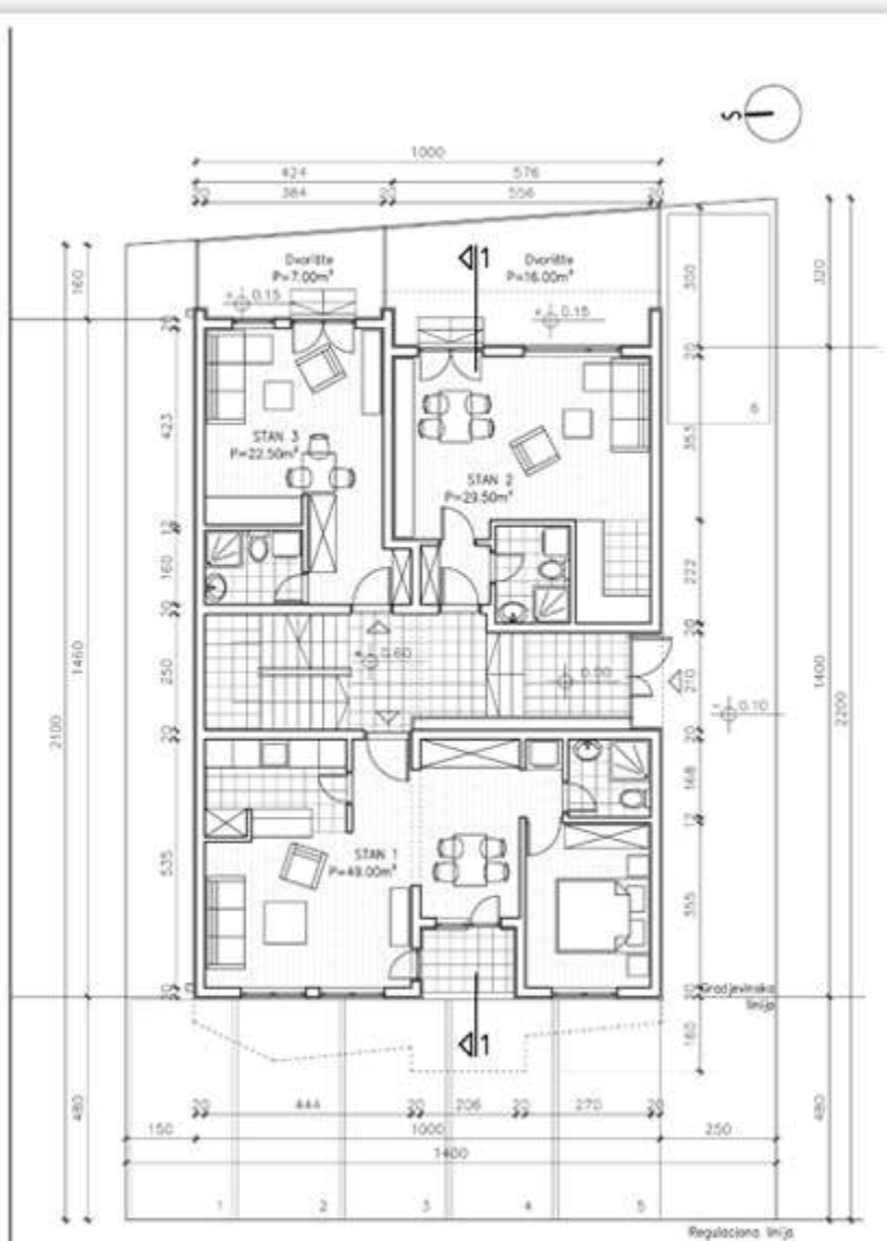
OSNOVA PRIZEMLJA 1:100
