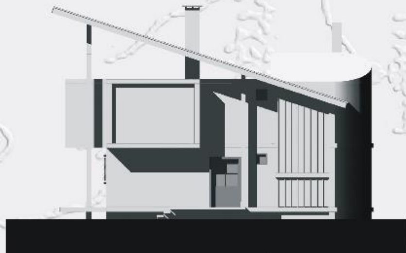
СЕВЕРОИСТОЧНА ФАСАДА R 1:100
