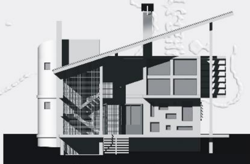
ЈУГОЗАПАДНА ФАСАДА R 1:100
