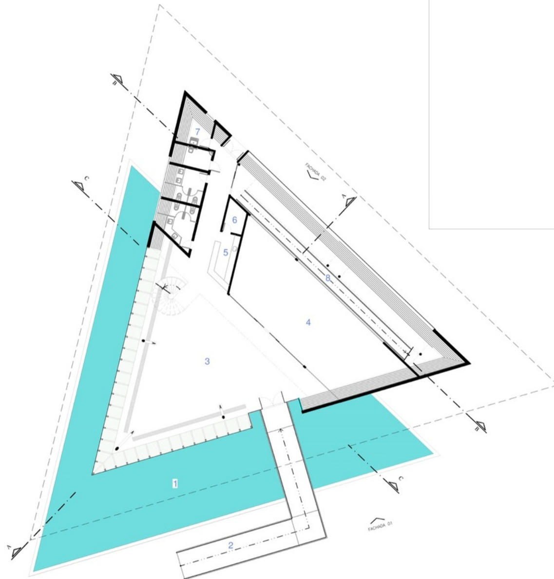
PLANTA-BAIXA / TÉRREO
