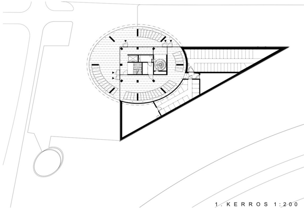
1. KERROS 1:200
