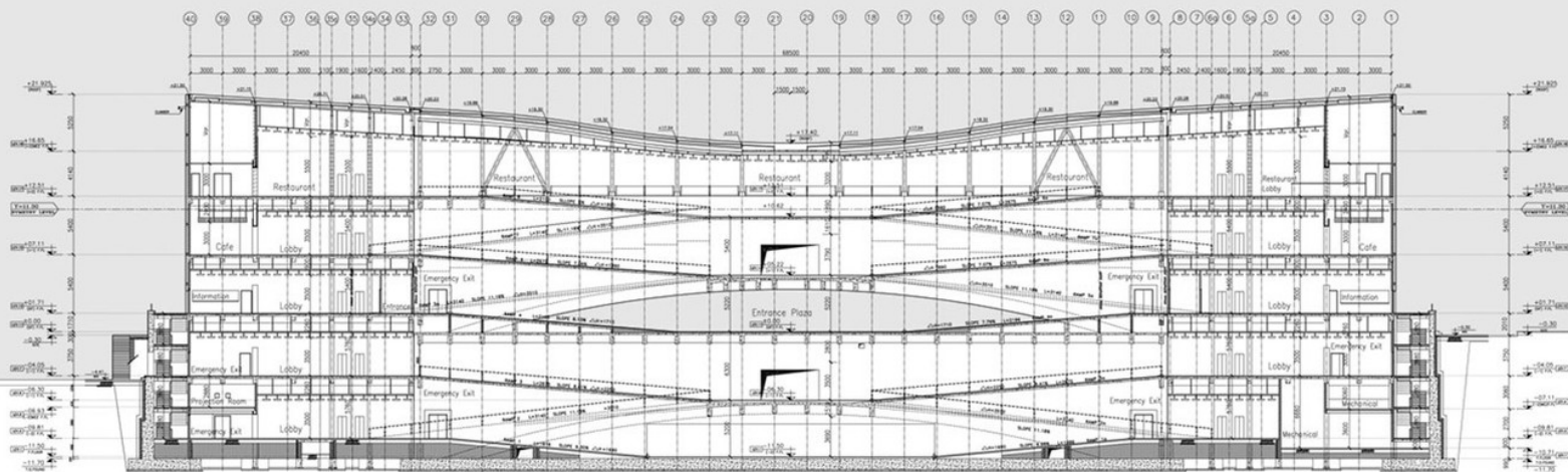
Longitudinal Section B-B SC / 1:600
